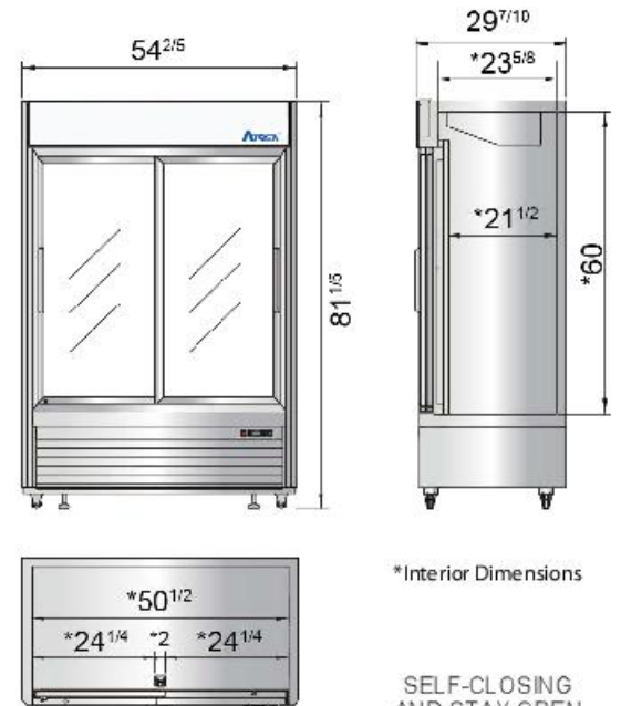
MCF8709GR
